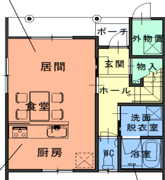
1階平面図
