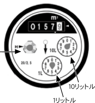
水道メーター
